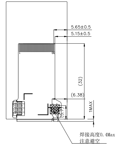
FPC弯折示意图 弯折出货
