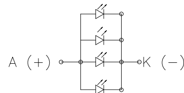
背光电路图(CIRCUIT DIAGRAM)
